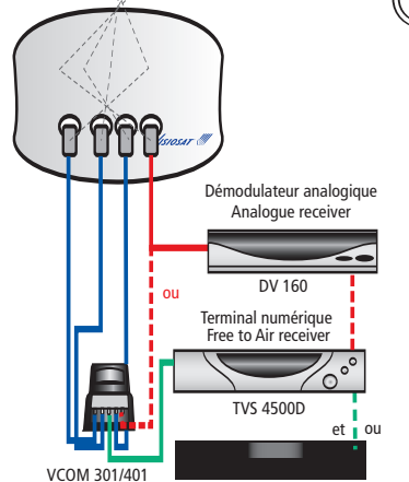
Terminal numérique à condition d'accès Digital receiver with conditionnal access
