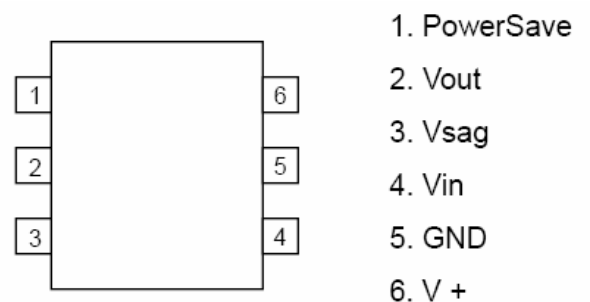
NJM2561F1; Vidio Amplifier (MTP6)
