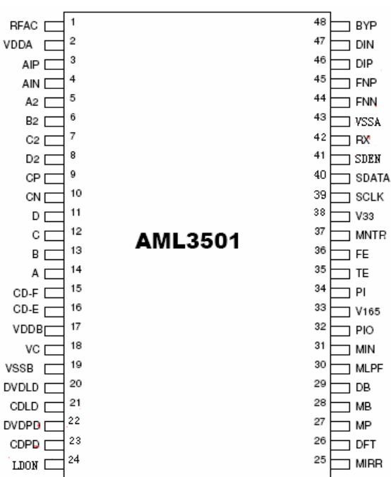
AML3501;DVD/CD RF Processor (TSSOP48)
