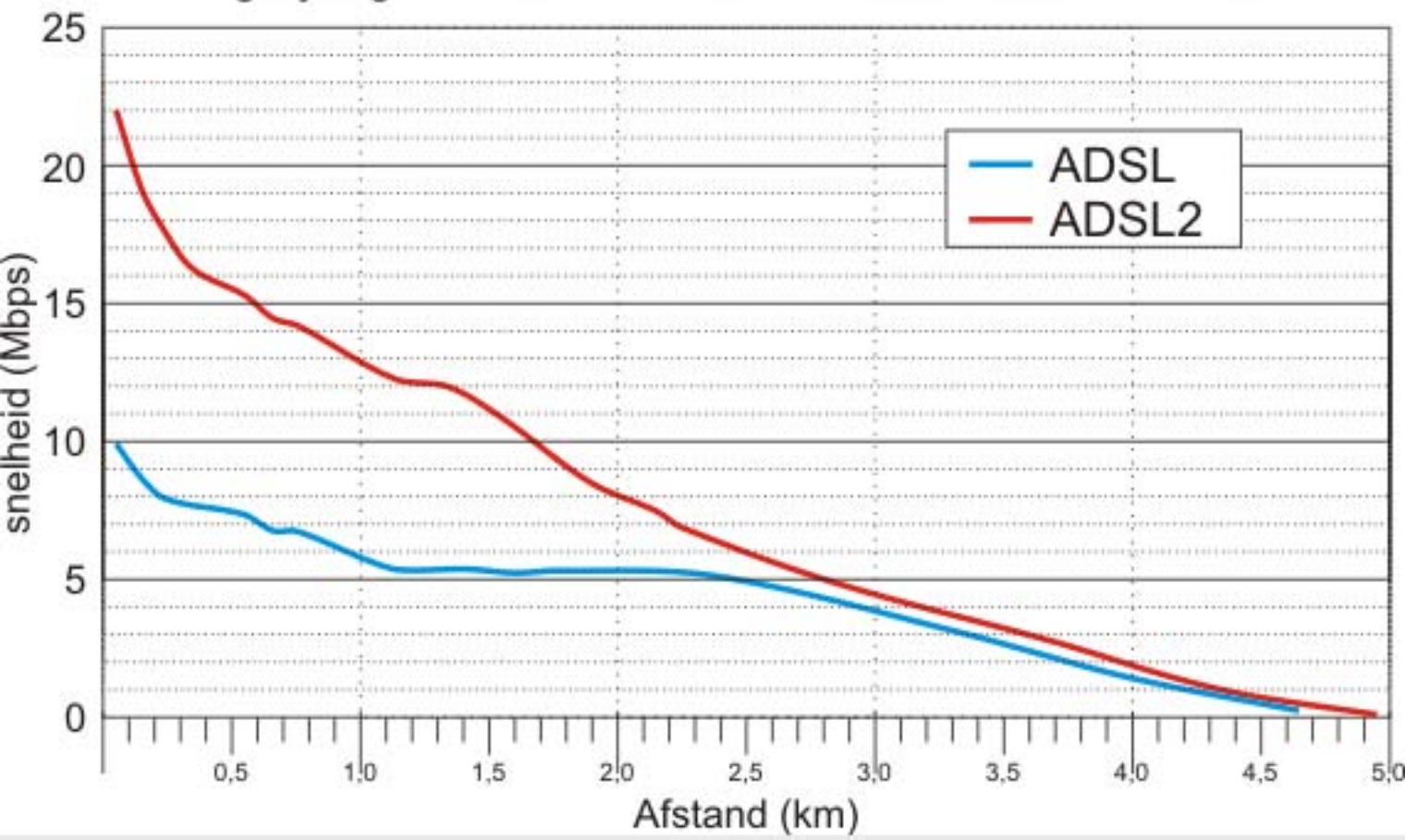
Vergelijking downstream snelheid tussen ADSL en ADSL2
