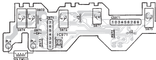
5 G MOTOR P.C.B. (REP2578A-N)
