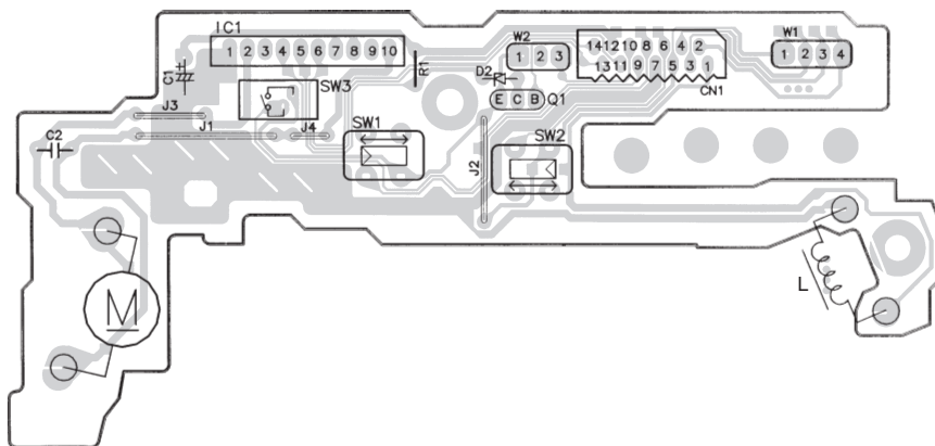
7 J TUNER PACK P.C.B. (REP1999B)
