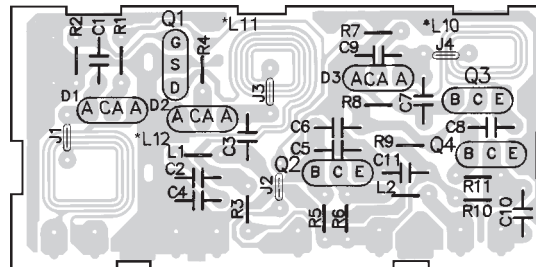
7 J TUNER PACK P.C.B. (REP1999B)
